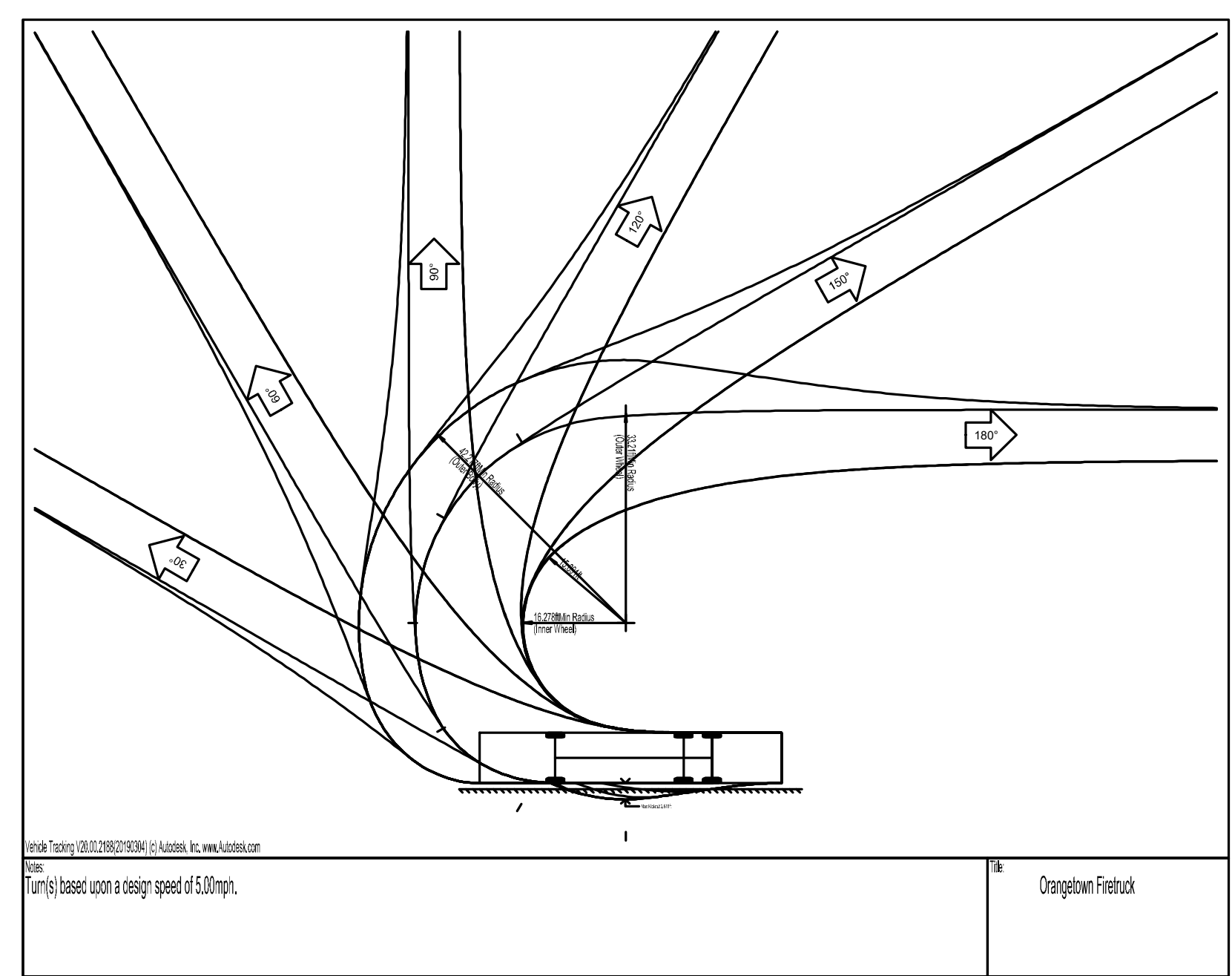
TURNING TEMPLATE SCALE: 1" = 20'
